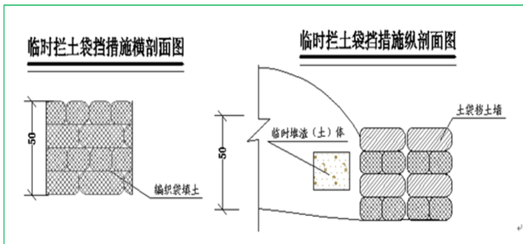
图 5-1 排土场临时挡土墙示意图
