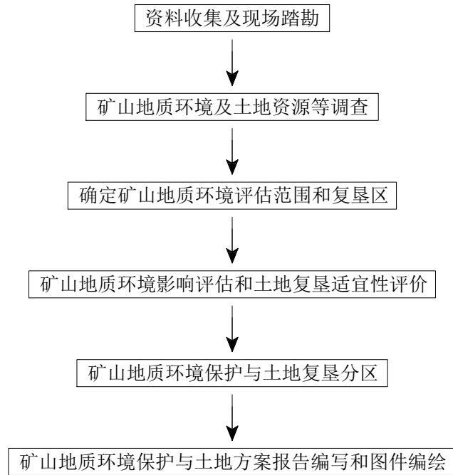
图 0-1 工作流程图
