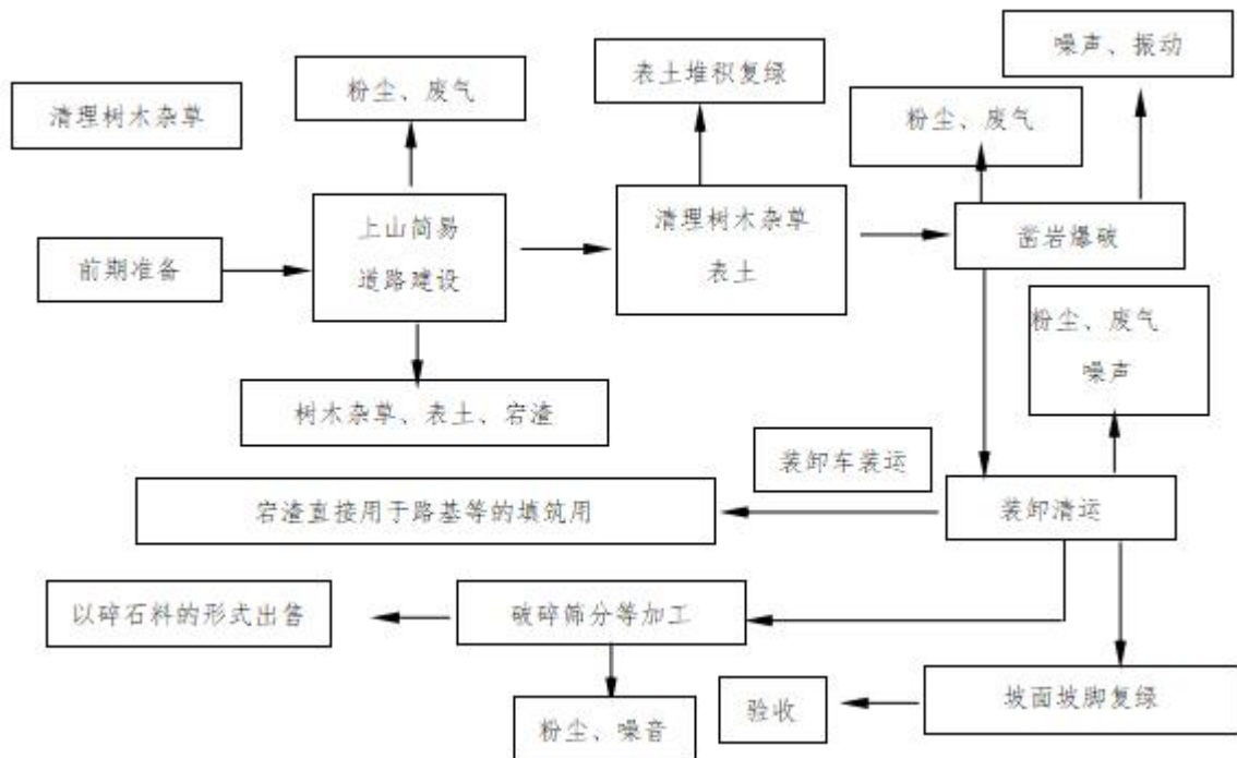
图 1-4 生产工艺流程图
