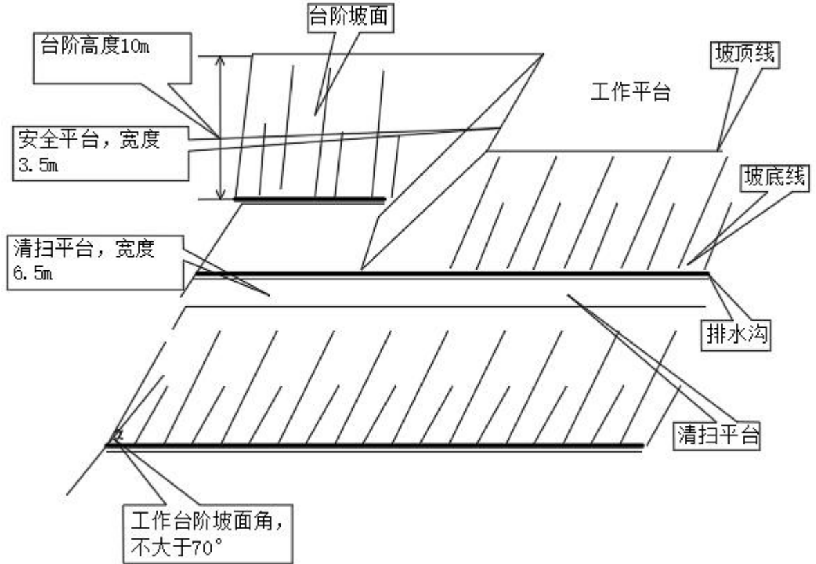
图 1-1 采矿方法标准图
