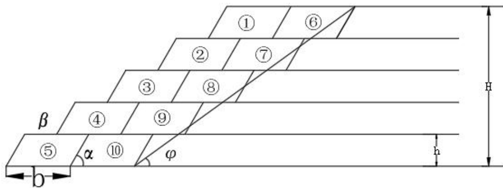
图 1-1 采矿方法标准图
