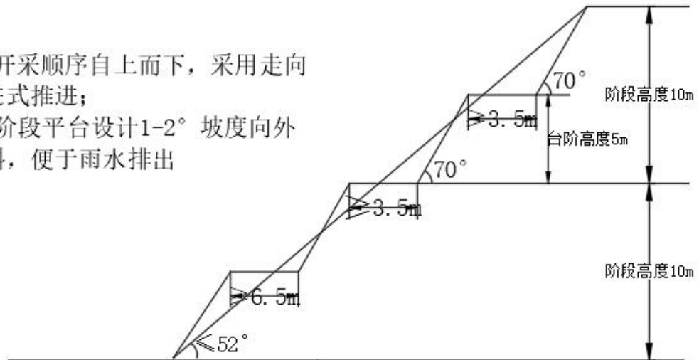
图 1-3 采矿方法剖面示意图
